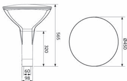
LEDPostTop-P D60
