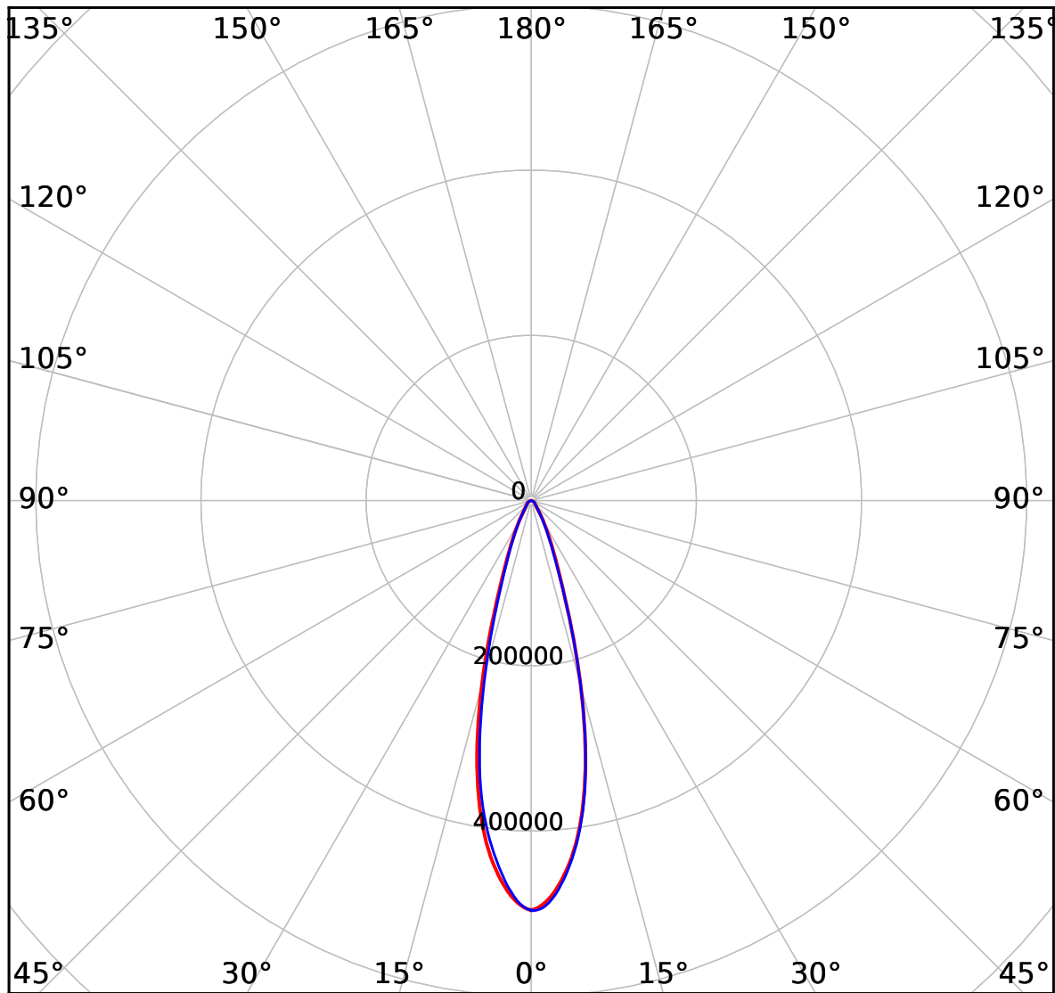
cd 160000 lm — C0-C180 — C90-C270
